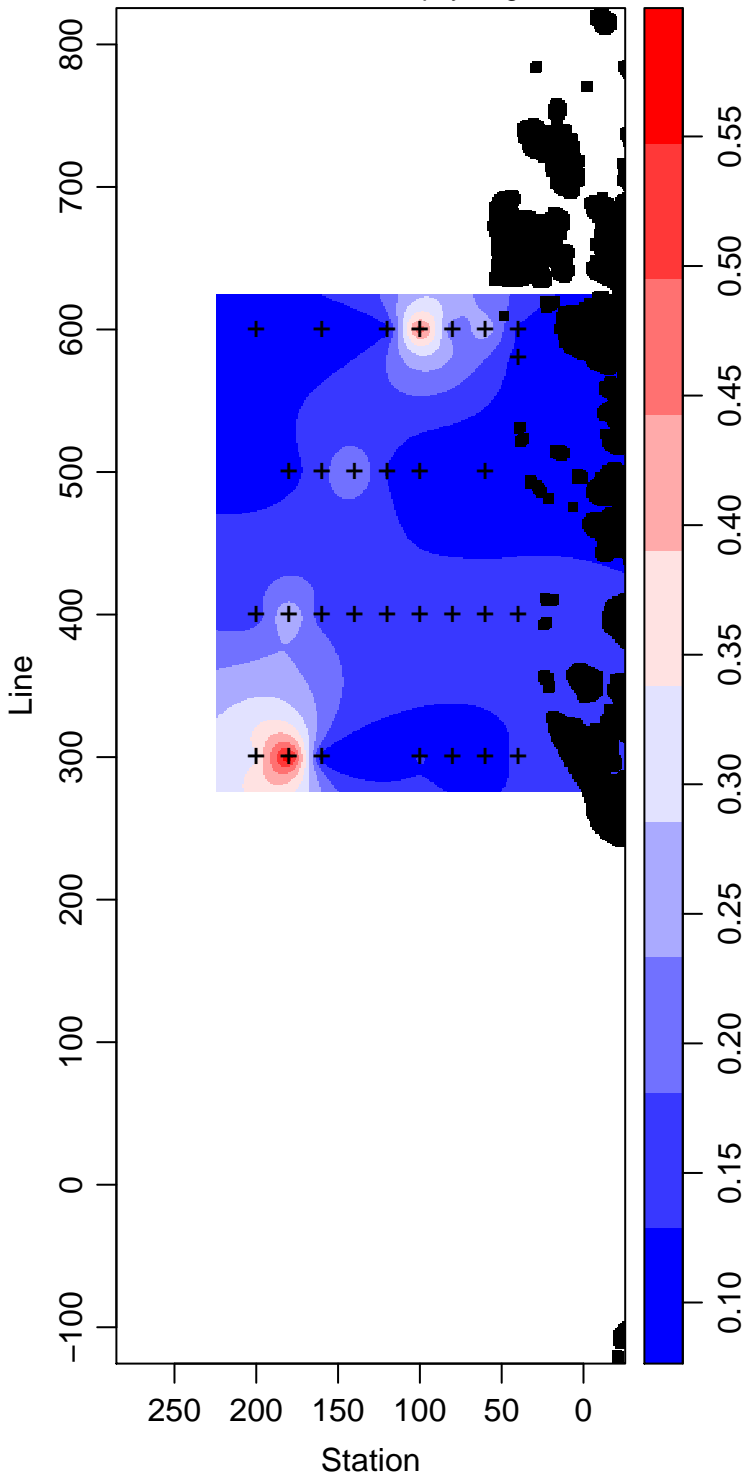
PD94-01_90_Chlorophyll mg m -3
