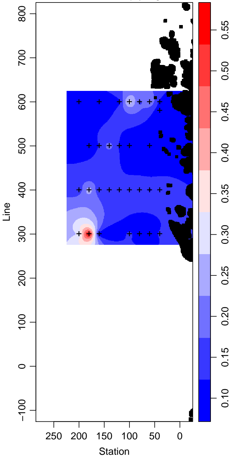
PD94-01_95_Chlorophyll mg m -3
