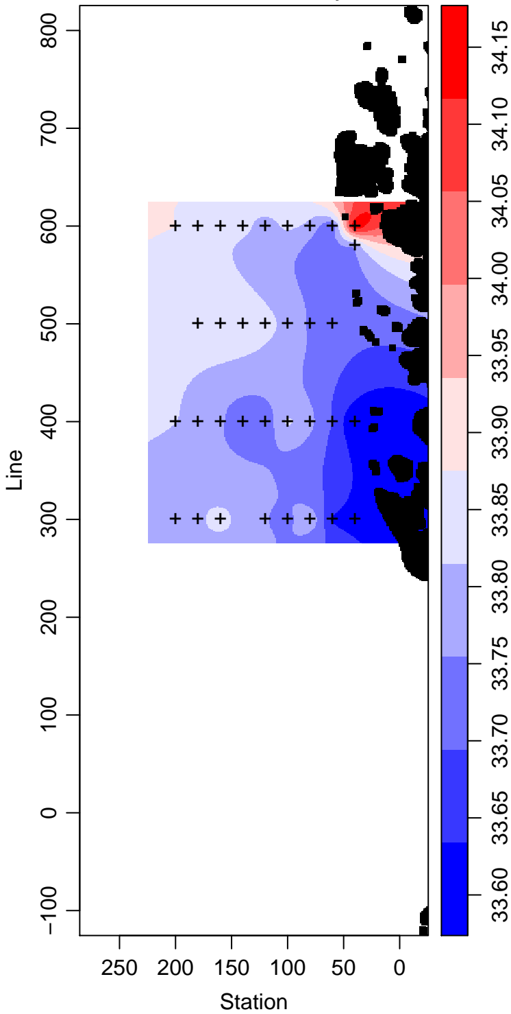
PD94-01_50_Salinity
