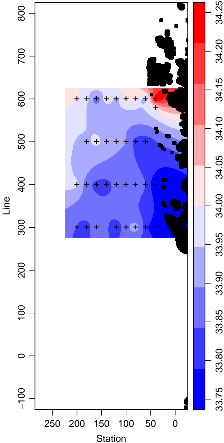
PD94-01_65_Salinity
