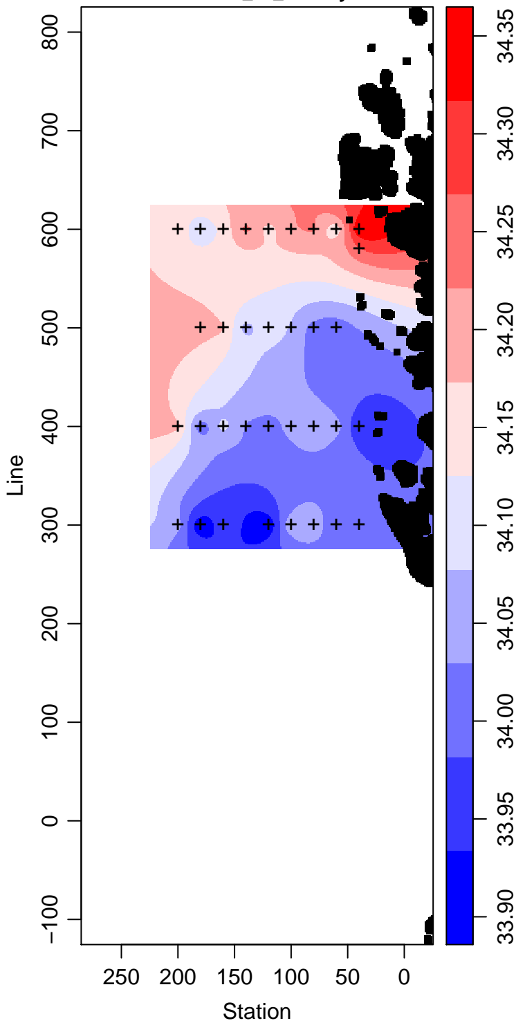
PD94-01_90_Salinity
