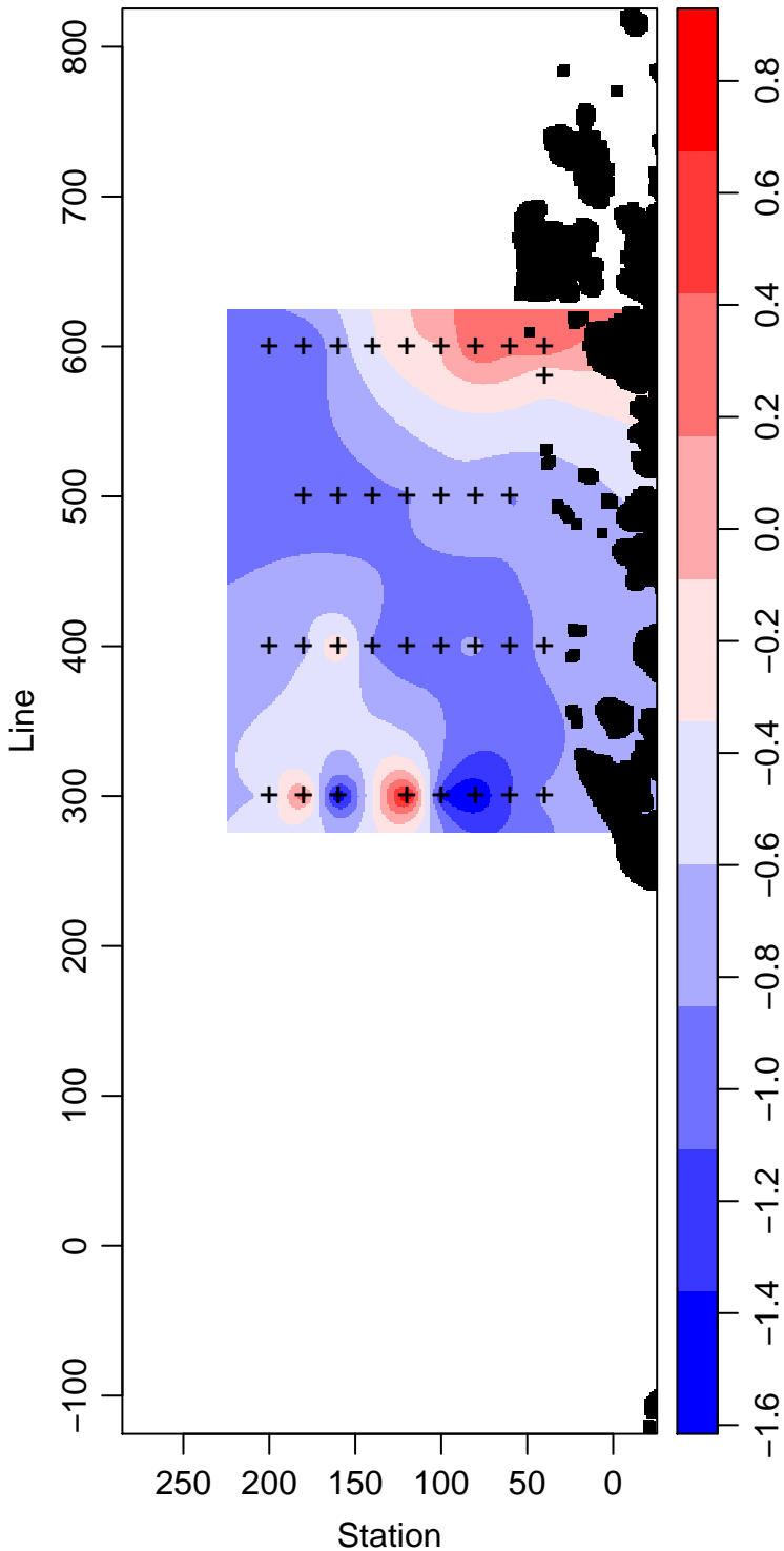
PD94-01_70_Temperature ° Celsius
