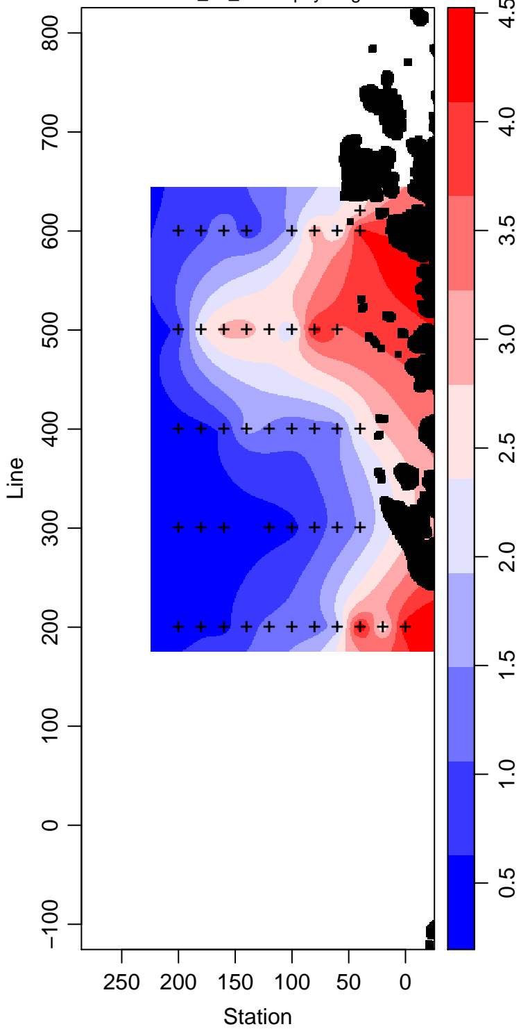
PD95-01_25_Chlorophyll mg m -3
