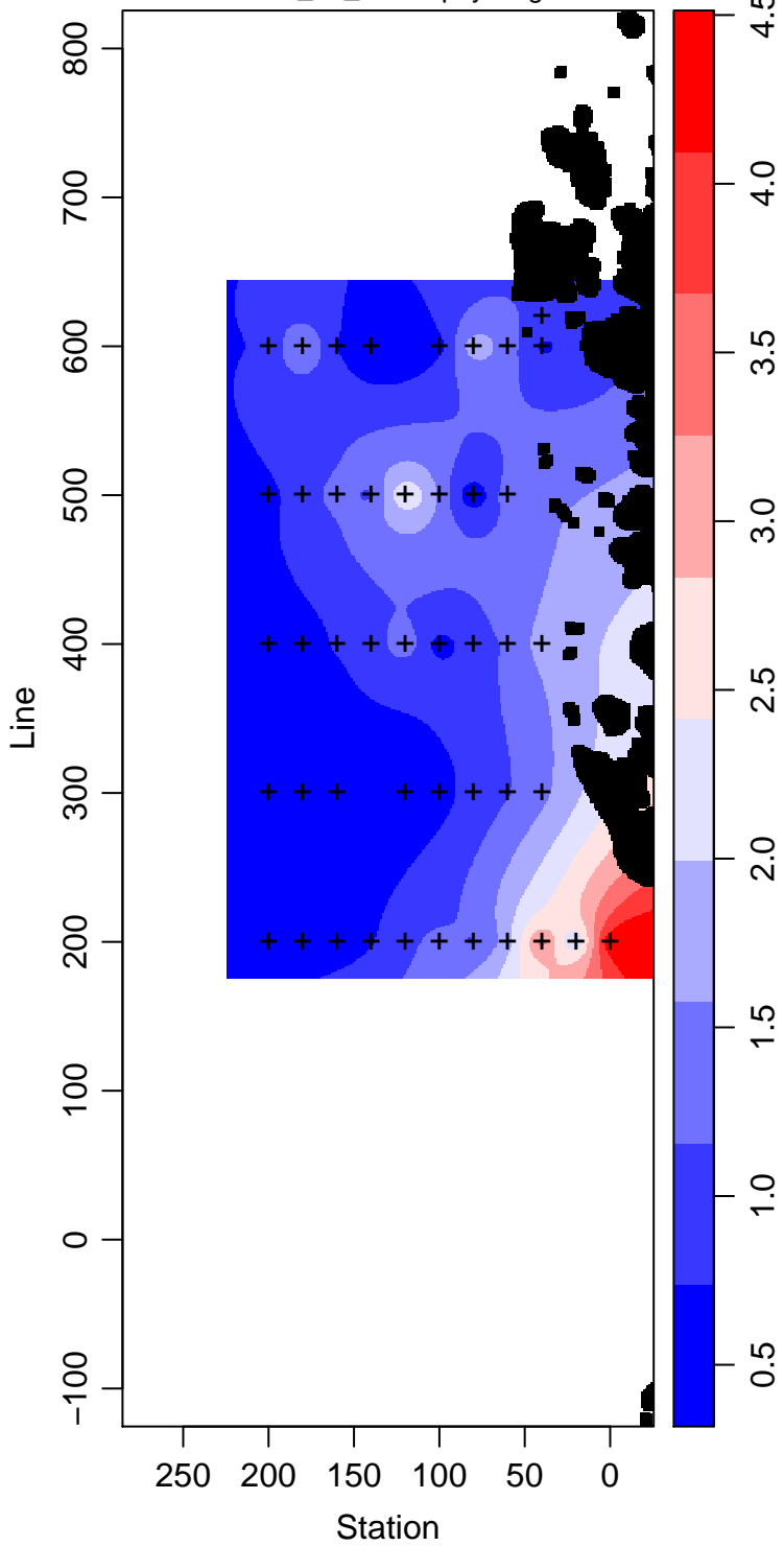
PD95-01_45_Chlorophyll \text{mg m}^{-3}
