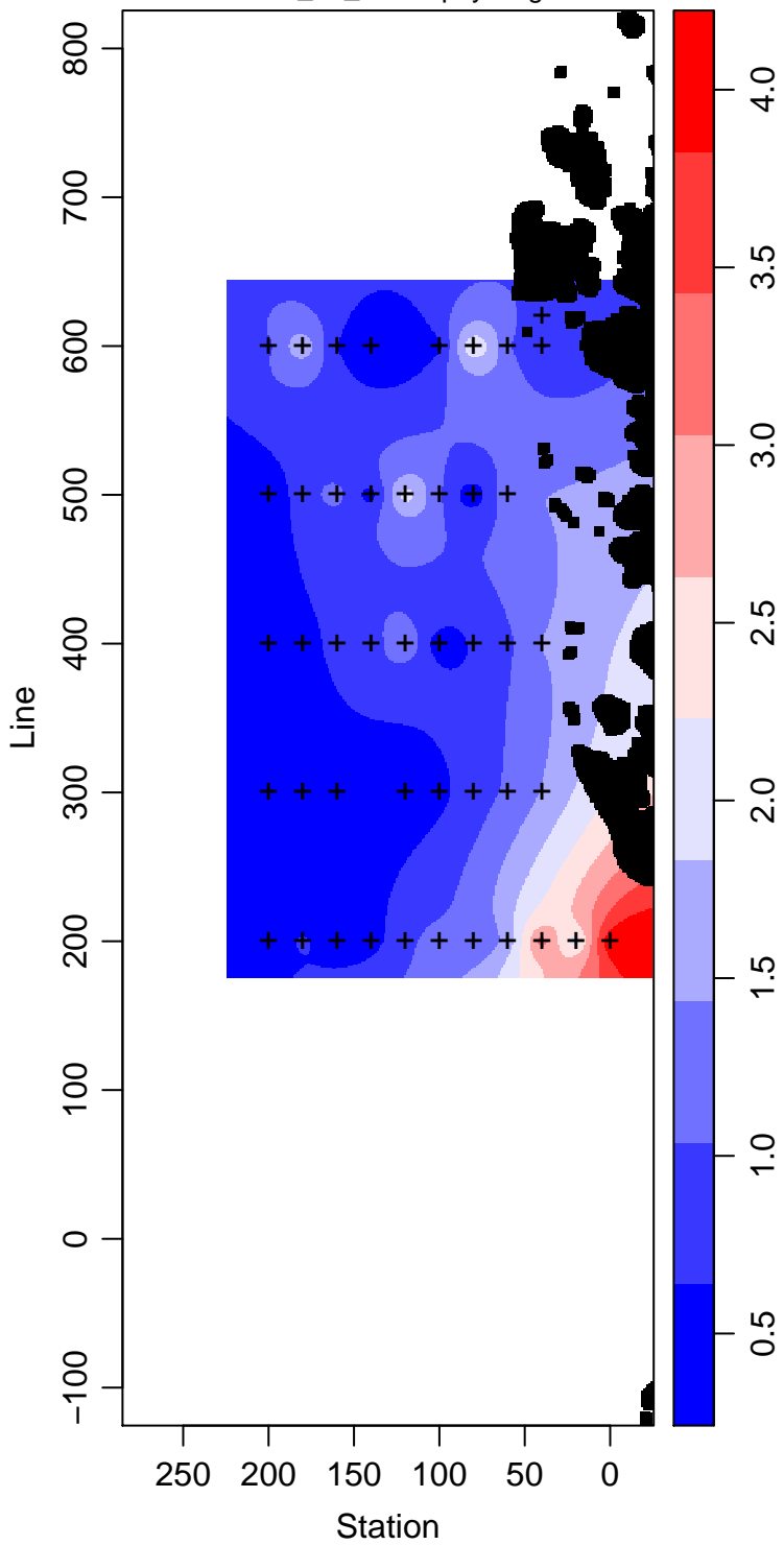
PD95-01_50_Chlorophyll mg m -3
