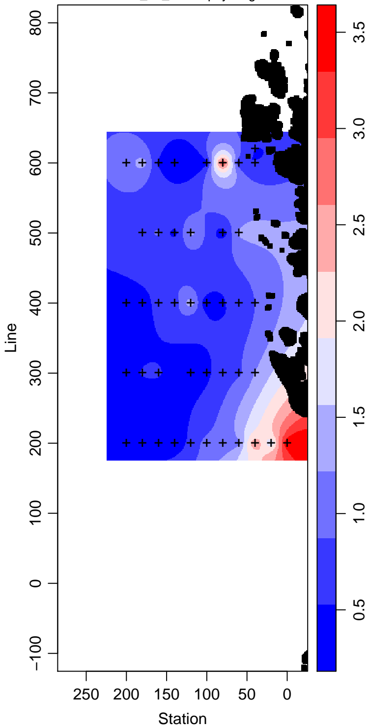
PD95-01_60_Chlorophyll mg m -3
