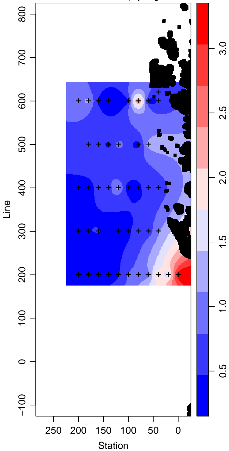
PD95-01_65_Chlorophyll mg m -3
