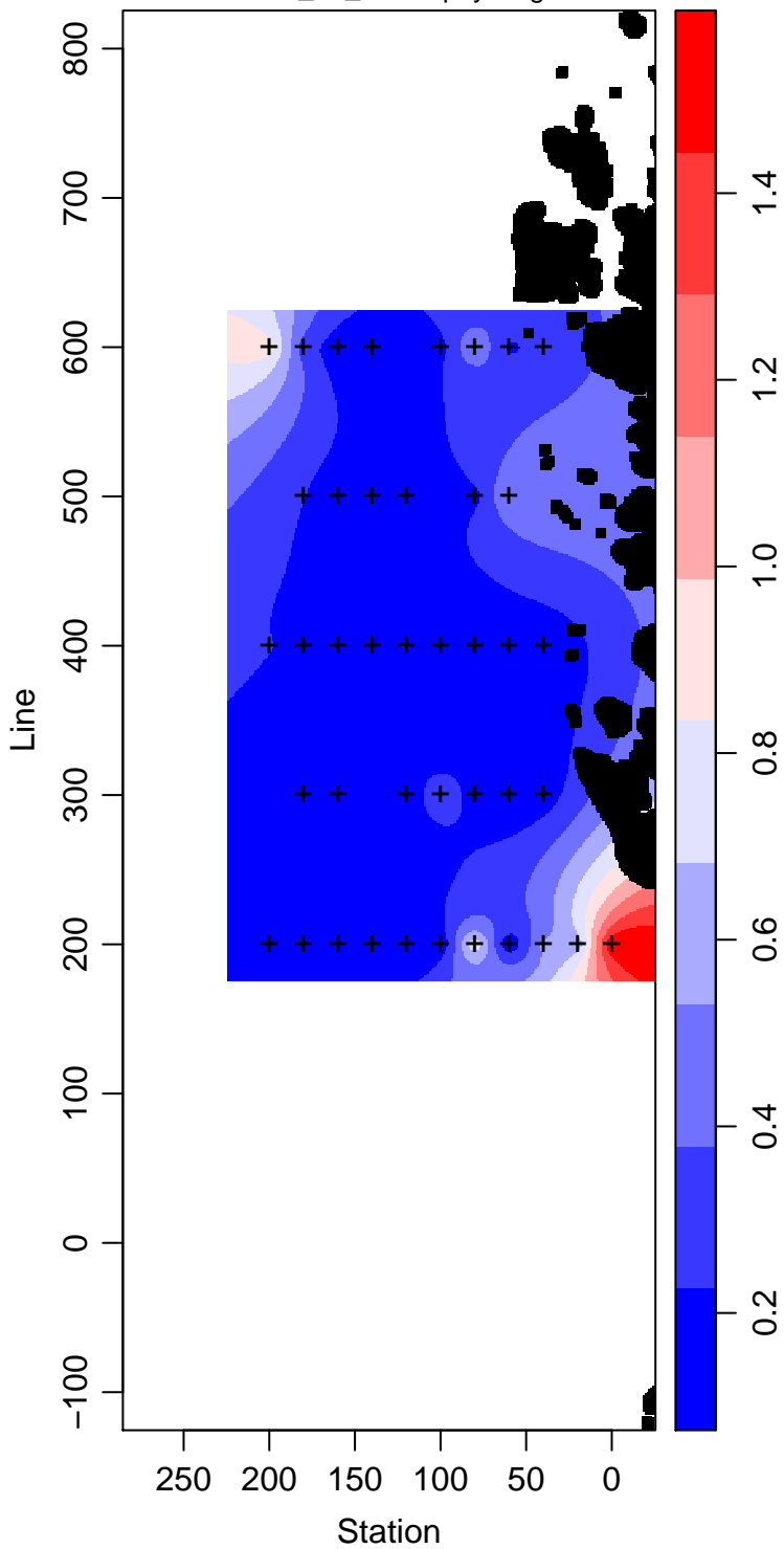
PD95-01_95_Chlorophyll mg m -3
