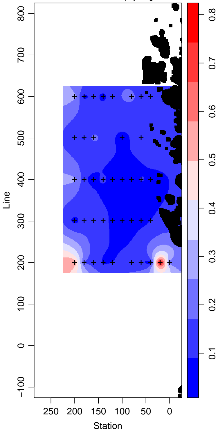
PD96-01_100_Chlorophyll \text{mg m}^{-3}
