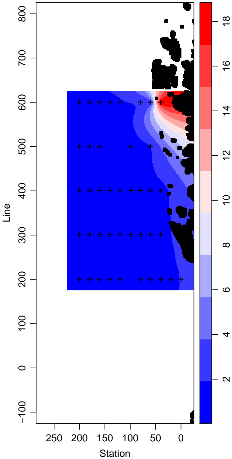
PD96-01_15_Chlorophyll mg m -3
