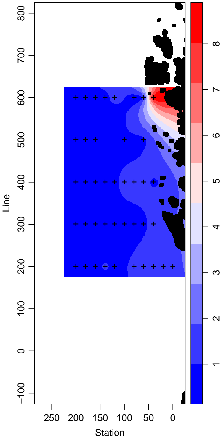
PD96-01_30_Chlorophyll mg m -3
