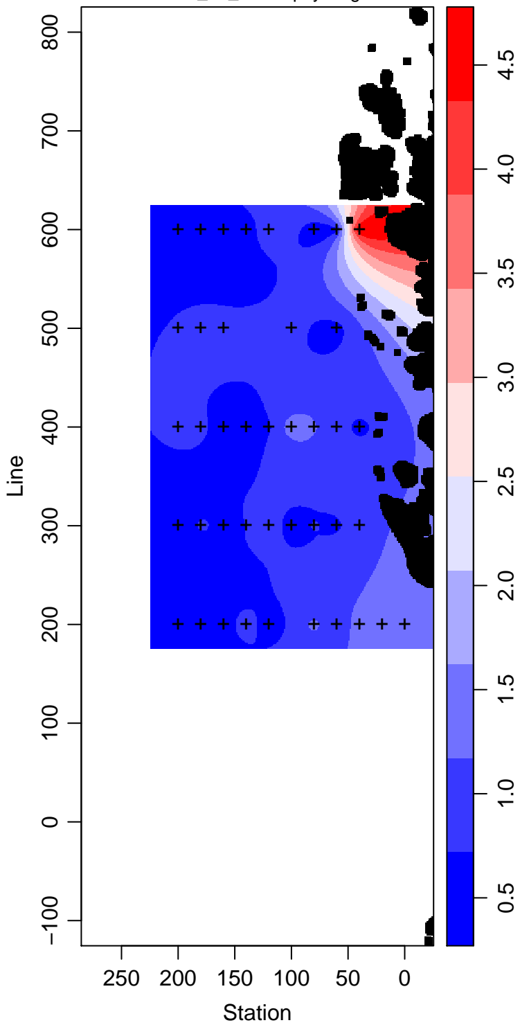
PD96-01_40_Chlorophyll mg m -3
