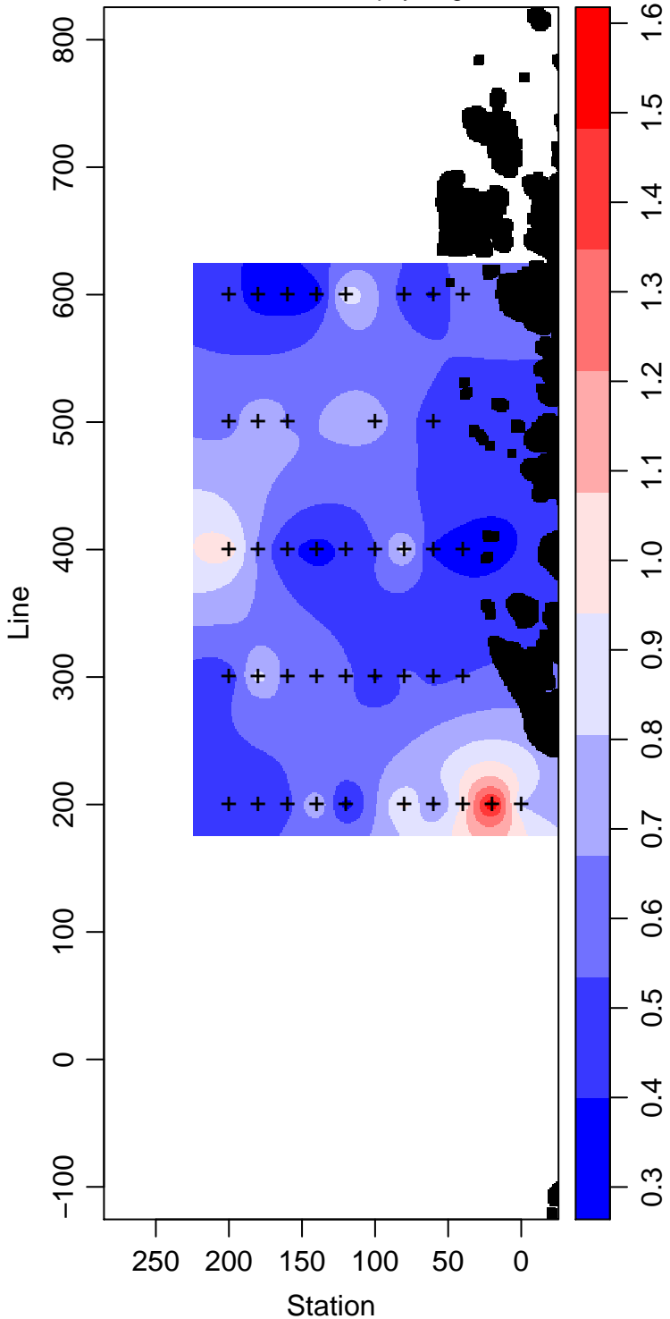
PD96-01_50_Chlorophyll mg m -3
