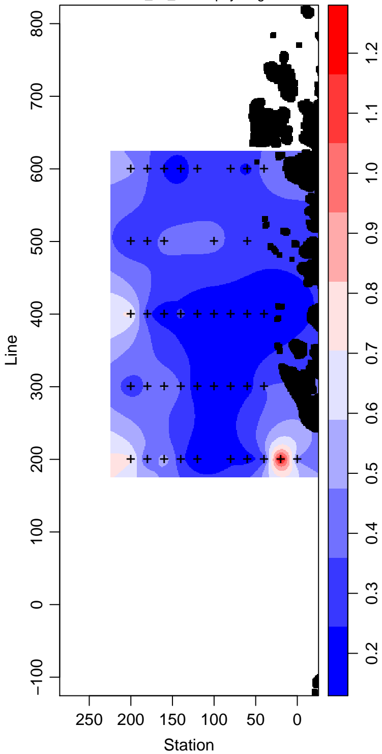
PD96-01_70_Chlorophyll mg m -3
