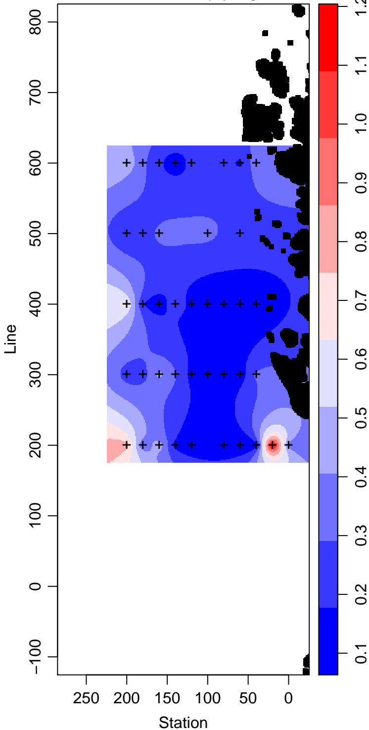
PD96-01_75_Chlorophyll \text{mg m}^{-3}
