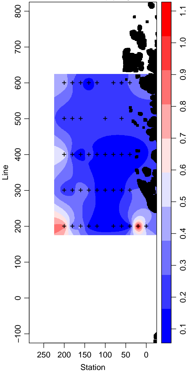
PD96-01_80_Chlorophyll mg m -3
