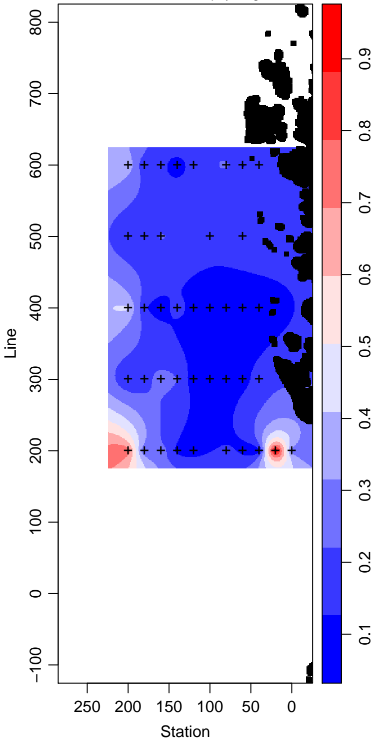
PD96-01_90_Chlorophyll mg m -3
