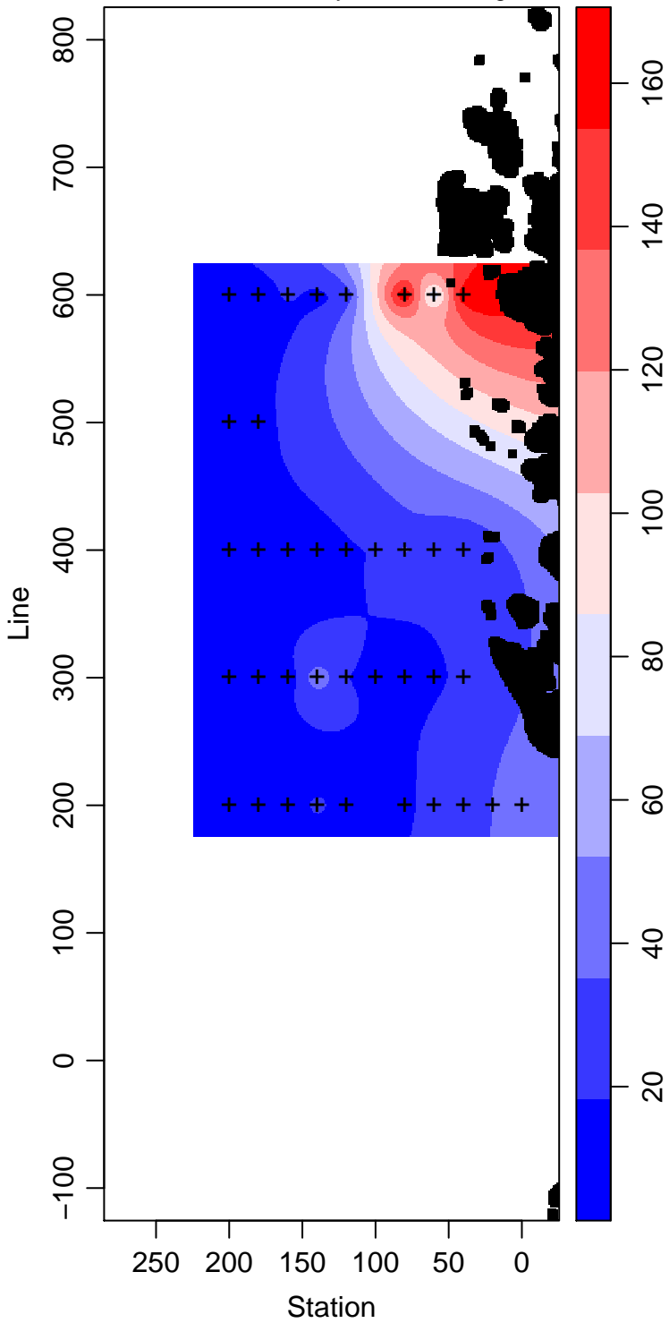
PD96-01_10_Primary.Production mg m -3
