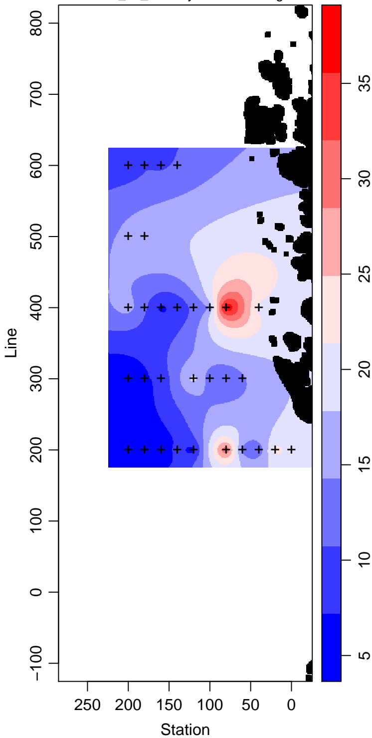
PD96-01_35_Primary.Production mg m -3
