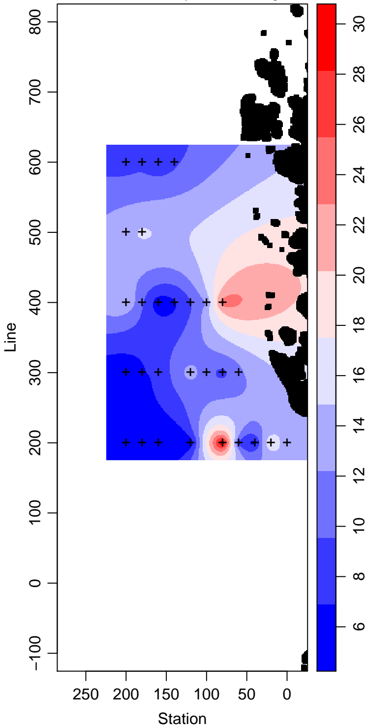
PD96-01_40_Primary.Production mg m -3
