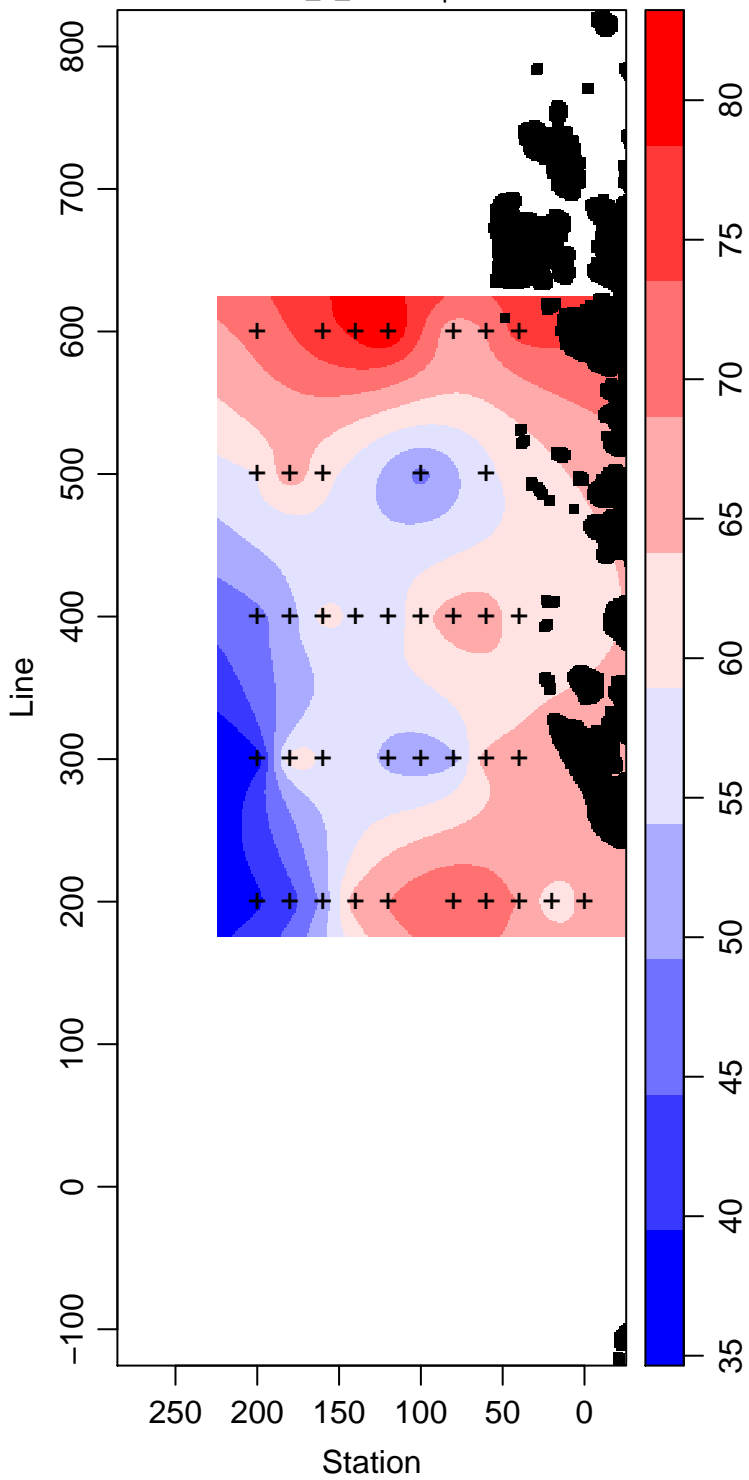
PD96-01_1_Silicate \mu\text{ mol L}^{-1}
