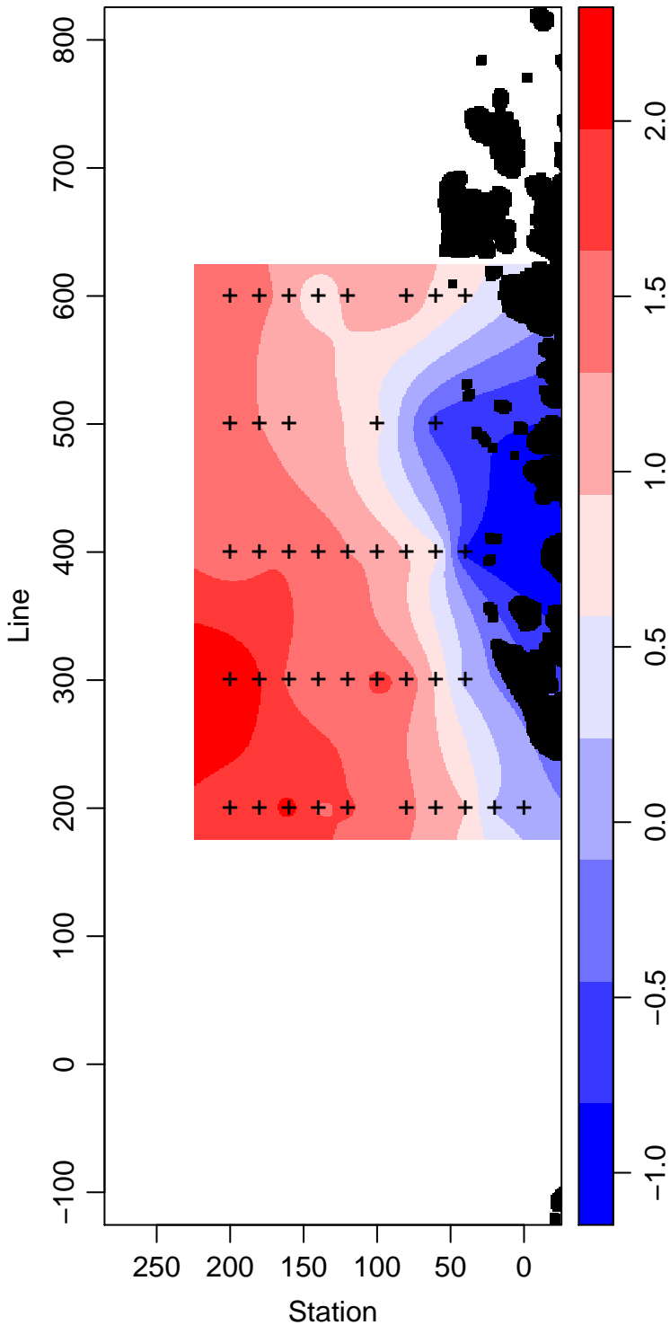
PD96-01_10_Temperature ° Celsius
