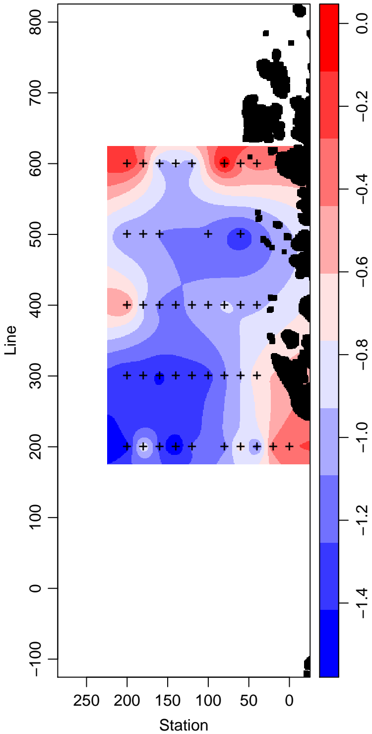
PD96-01_70_Temperature ° Celsius
